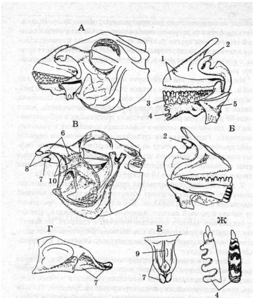
Рис. 1. Особенности строения челюстного аппарата лоры. А — череп лоры \times 1,5 , В — челюсти: а) снаружи, б) изнутри, В — щечный отдел, Г — обонятельно-сошниковый блок (сбоку), Е — то же (сверху), Ж — симфиз нижней челюсти, форма сочленовных зубчиков. Кости черепа: 1 — зубная пластинка верхней челюсти; 2 — сочленовный отросток верхней челюсти; 3 — зубная пластинка нижней челюсти; 4 — шов снаружи и форма зубчиков; 5 — сочленовная; 6 — небная; 7 — сошник; 8 — сочленовные поверхности небной и сошника; 9 — среднеобонятельная; 10 — крыловидные.
